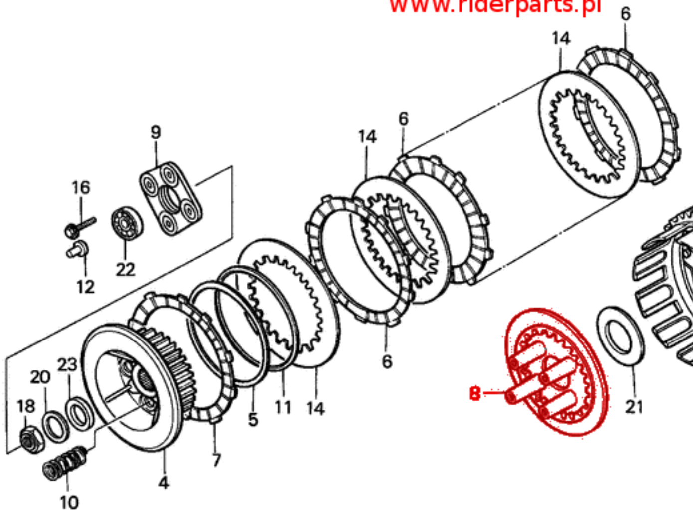
Schemat: Honda XL600V Transalp PD1
